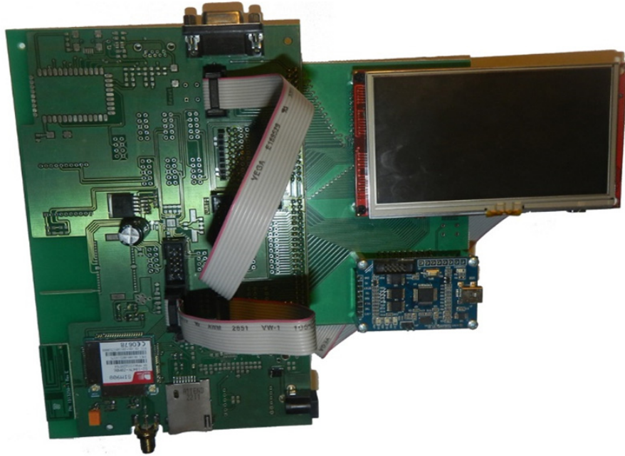
Fig. 1-1 DSPLABS_DT_STK_V1
